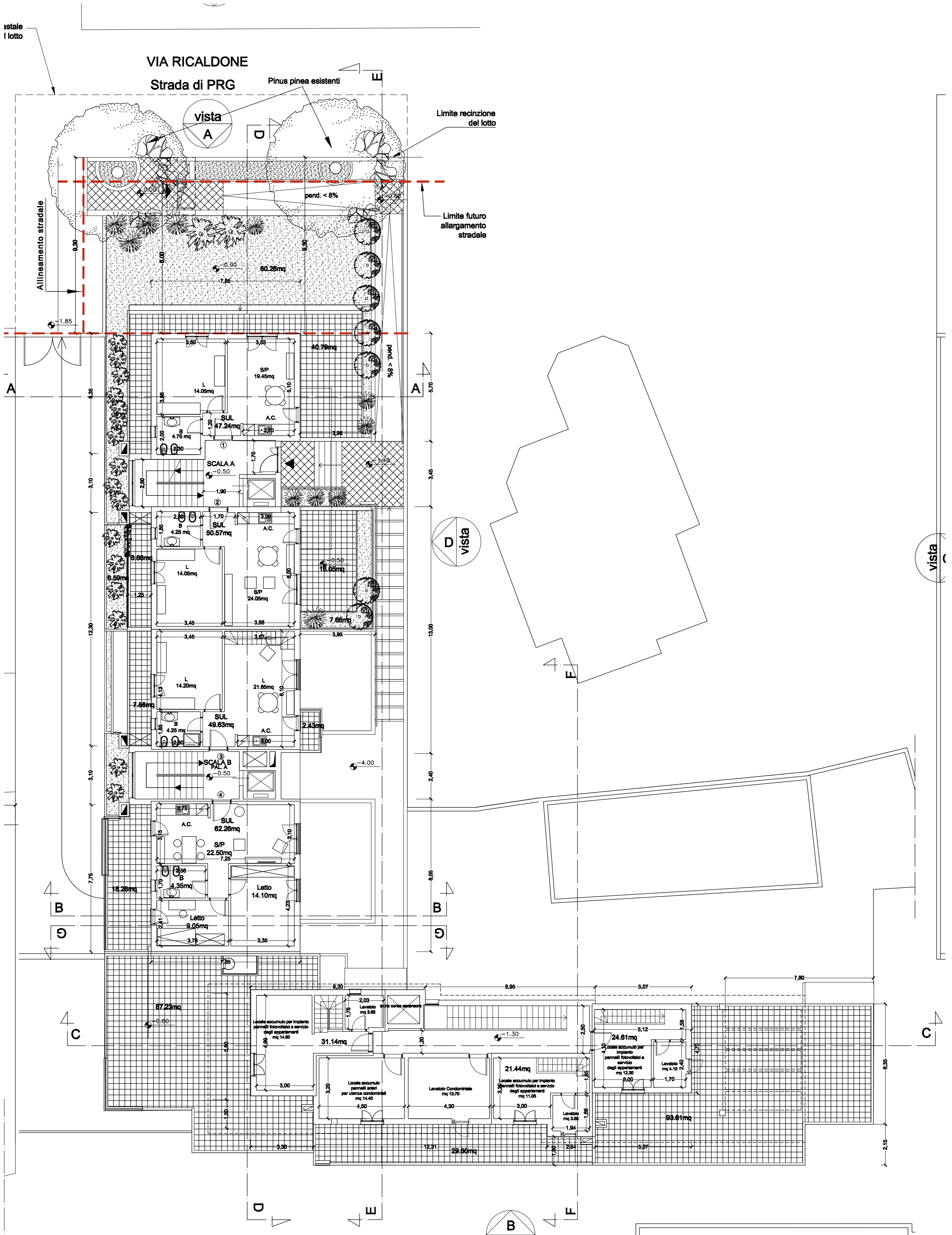
PIANO PRIMO PAL. A / PIANO SECONDO PAL. B Rapp. 1:100
